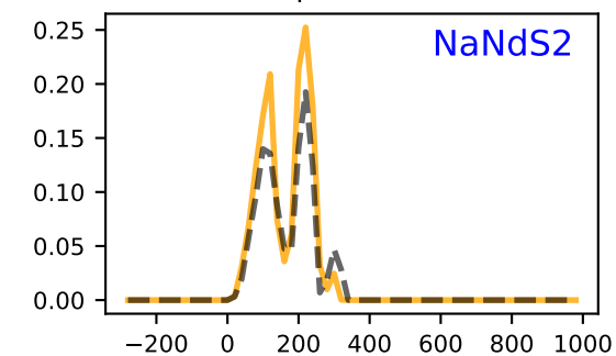
mp-675562
