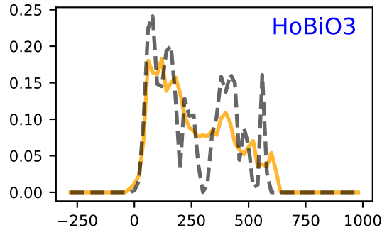
mp-770830
