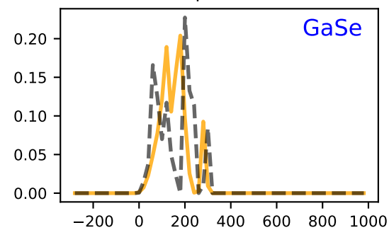
mp-1572
