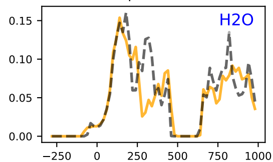
mp-31117
