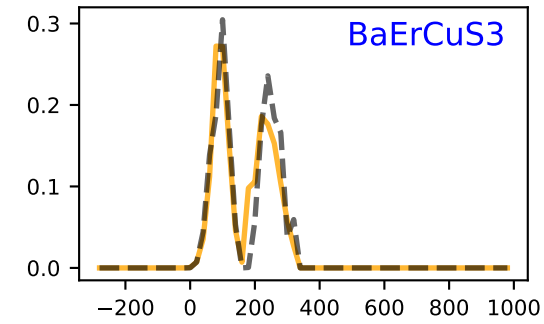
mp-14969
