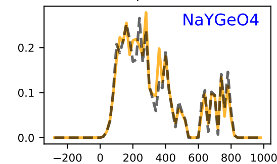
mp-17394
