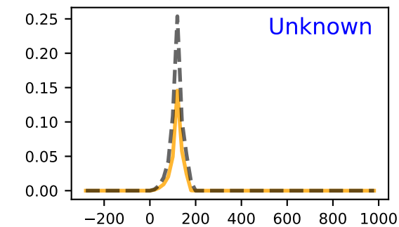
JVASP-3162
