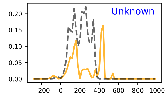
mp-769971
