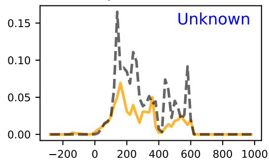
mp-35421
