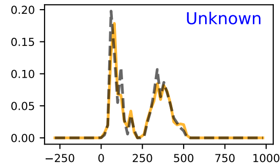
JVASP-26396
