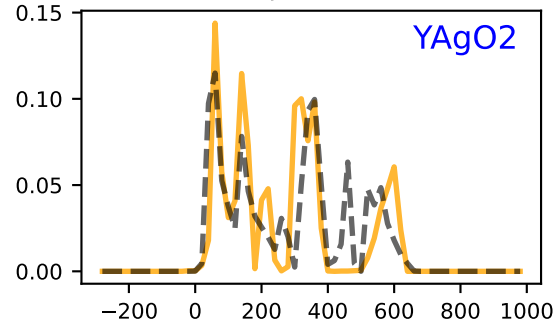
JVASP-16563
