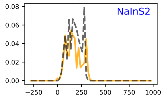
JVASP-12591
